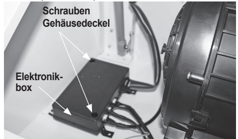
Abb. 6a (Abb. ähnlich)
