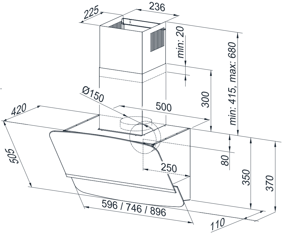
Abb. 18 Abmessungen Modelle „Rota“
