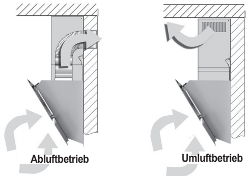
Abb. 7 (Abb. ähnlich; Prinzipdarstellung) Abb. 8
